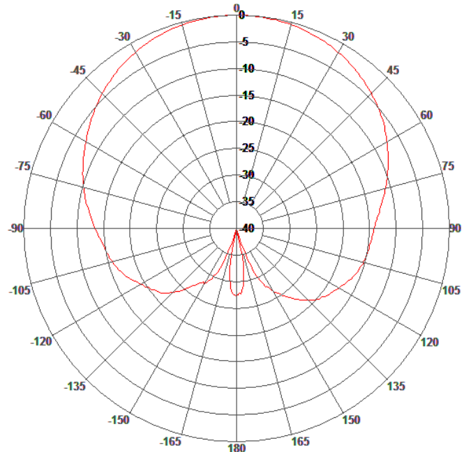
H-Plane Patterns
