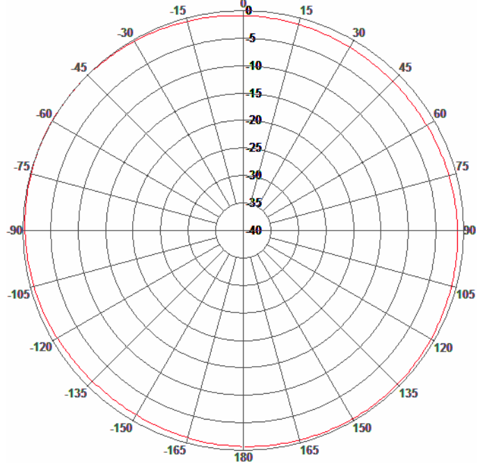
H-Plane Pattern
