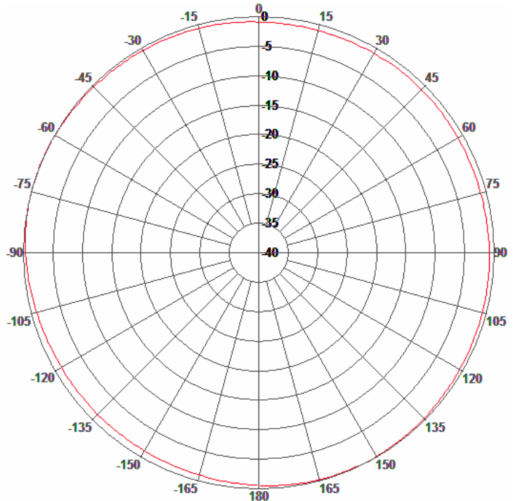
H-Plane Pattern
