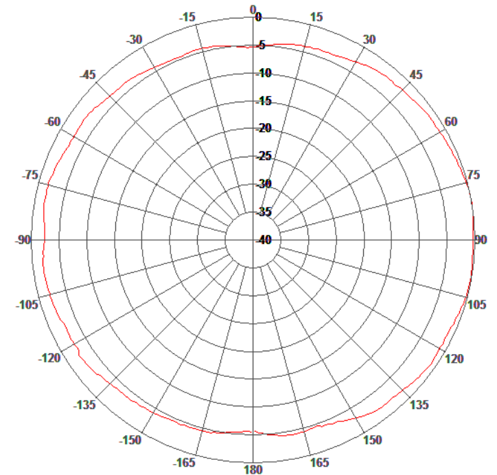
H-Plane Pattern
