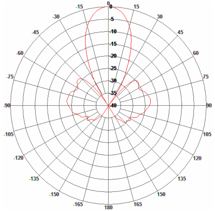
H-Plane Pattern
