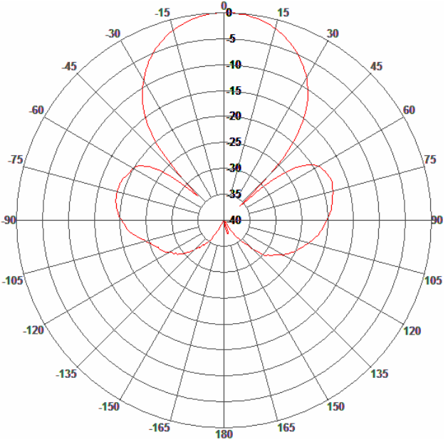
H-Plane Pattern
