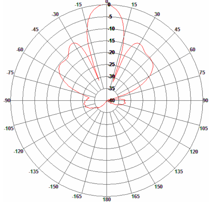
H-Plane Pattern
