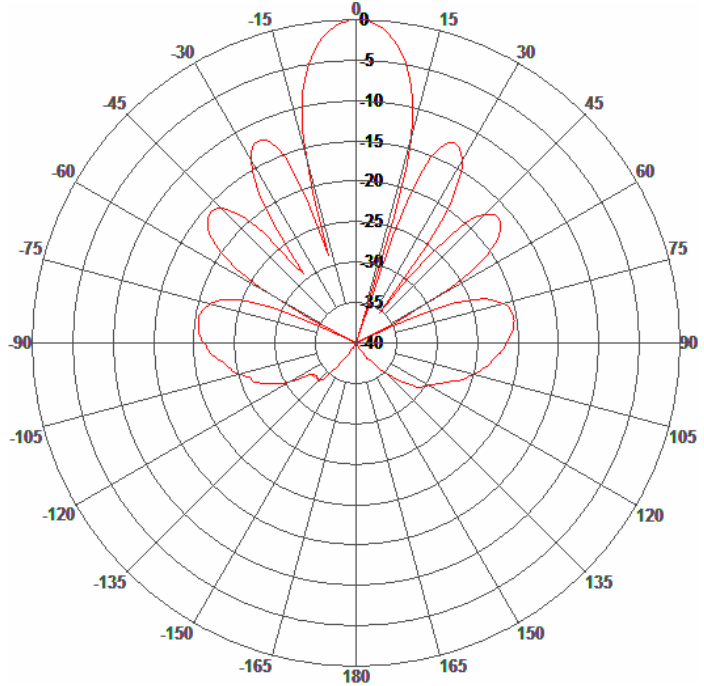
H-Plane Pattern
