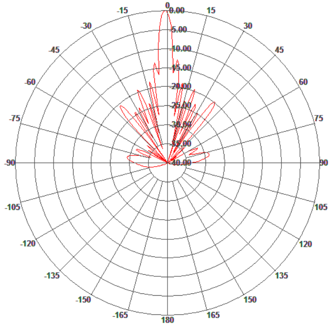
H-Plane Pattern
