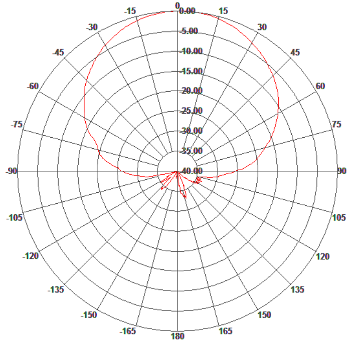
H-Plane Patterns
