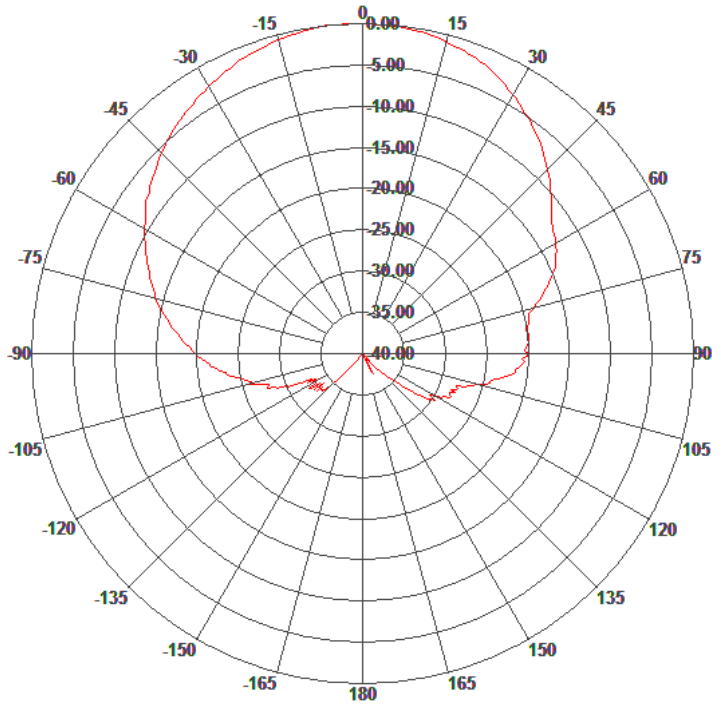
H-Plane Pattern
