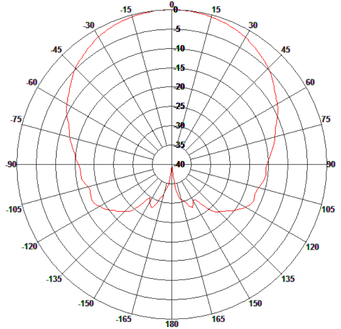
H-Plane Patterns
