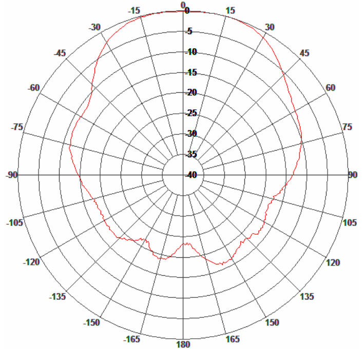
H-Plane Pattern
