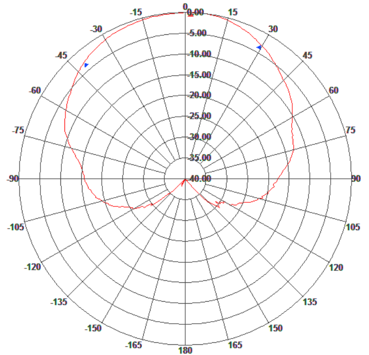
H-Plane Pattern
