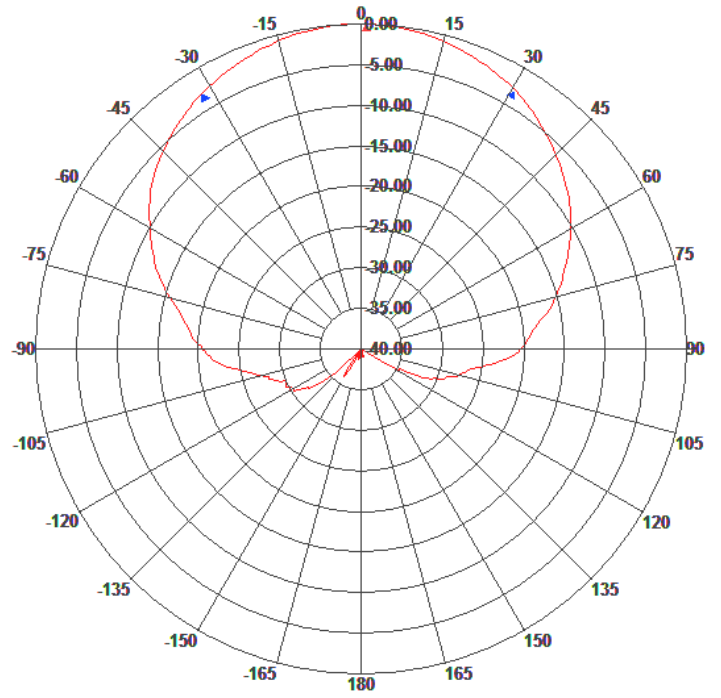
H-Plane Patterns
