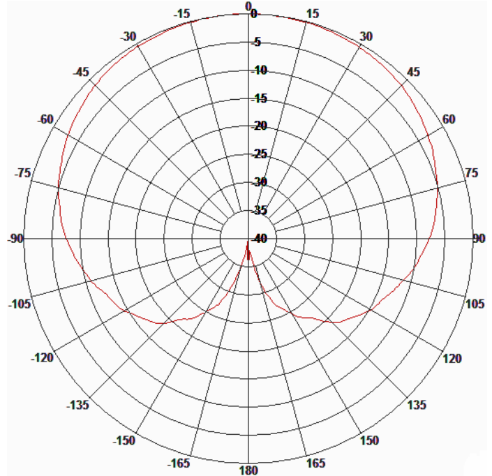
H-Plane Pattern
