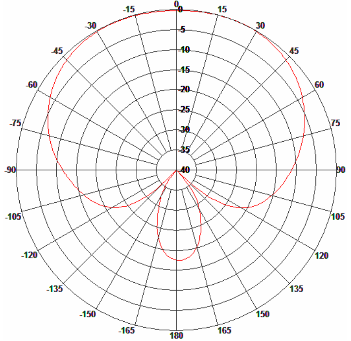
H-Plane Patterns
