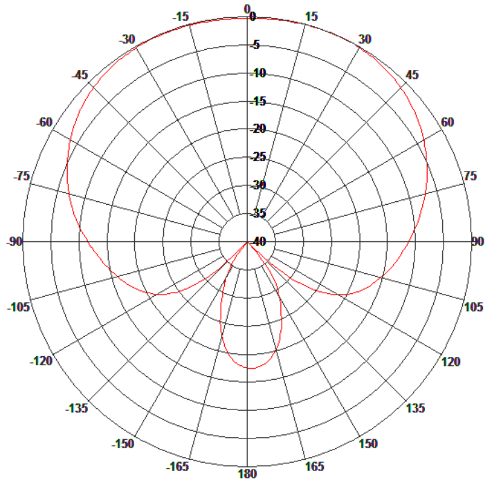
H-Plane Patterns
