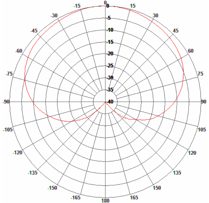
H-Plane Pattern
