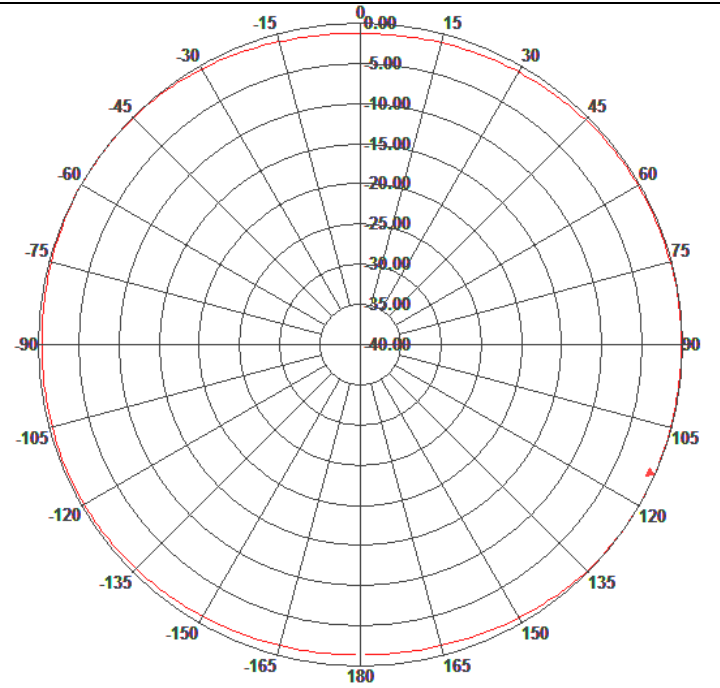
H-Plane Pattern
