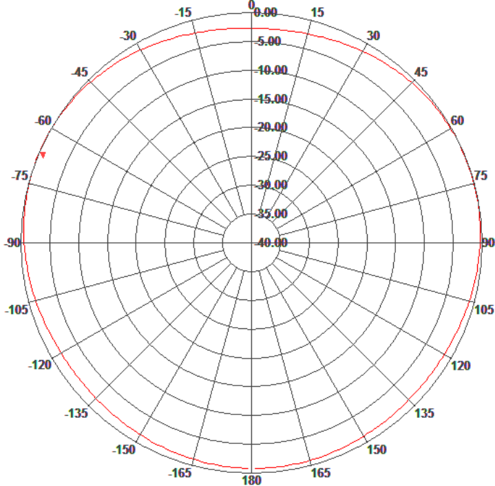
H-Plane Pattern
