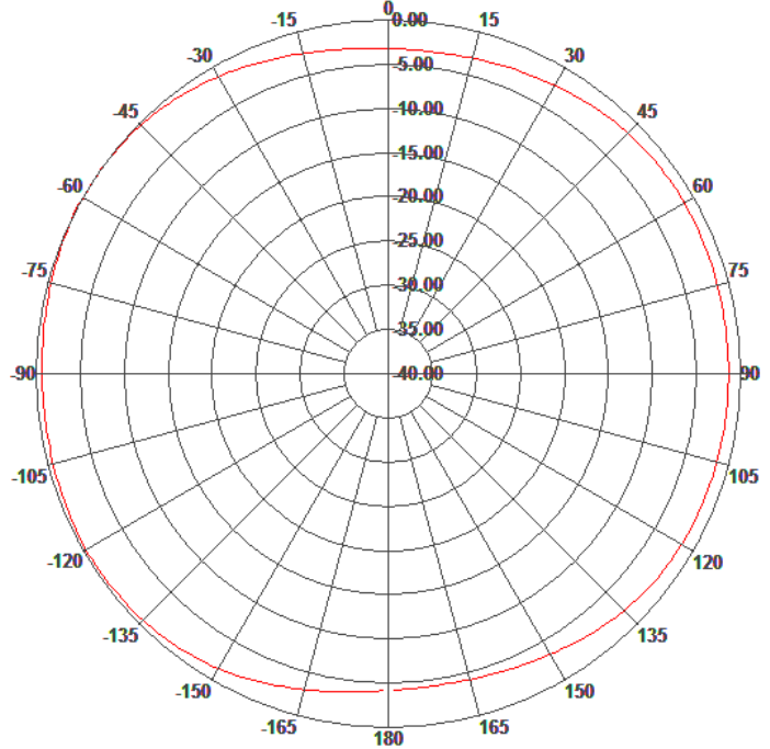
H-Plane Patterns
