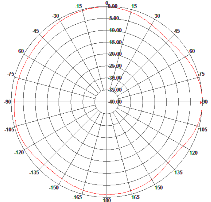
H-Plane Pattern
