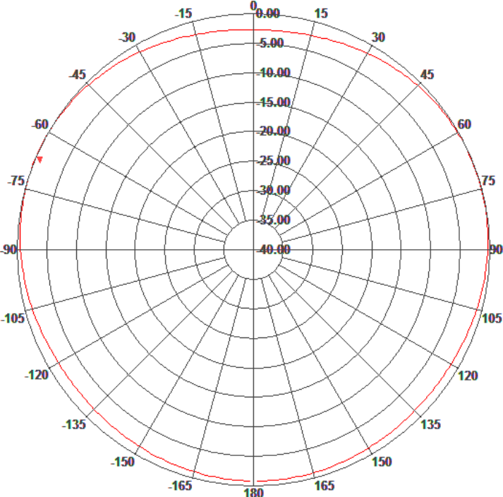
H-Plane Pattern
